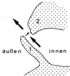
Abb. 2. Querschnitt der äußeren Riechsacköffnung (schematisch bei Offenstellung des Hautlappens (1). 2, dorsaler Rand der Öffnung.
